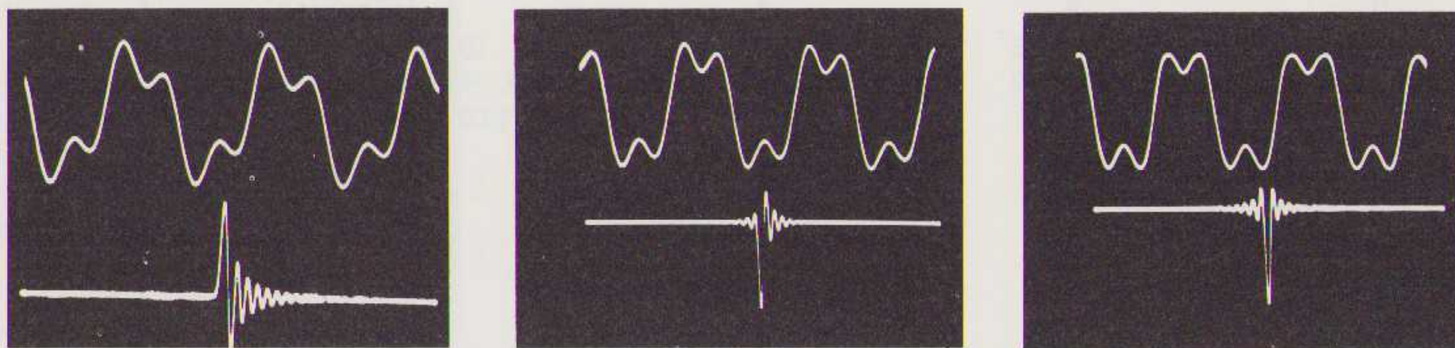
Blokgolfbeelden bij 5 kHz (boven) en naaldimpulsweergave (onder) bij de drie thans voorkomende spelertypes met resp. 16 bit lineaire D/A omzetting en analoge filtering (links), 16 bit 2-voudige oversampling en digitaal/analoge filtering (mid-den) en 14 bit 4-voudige oversampling en digitaal/analoge filtering.
